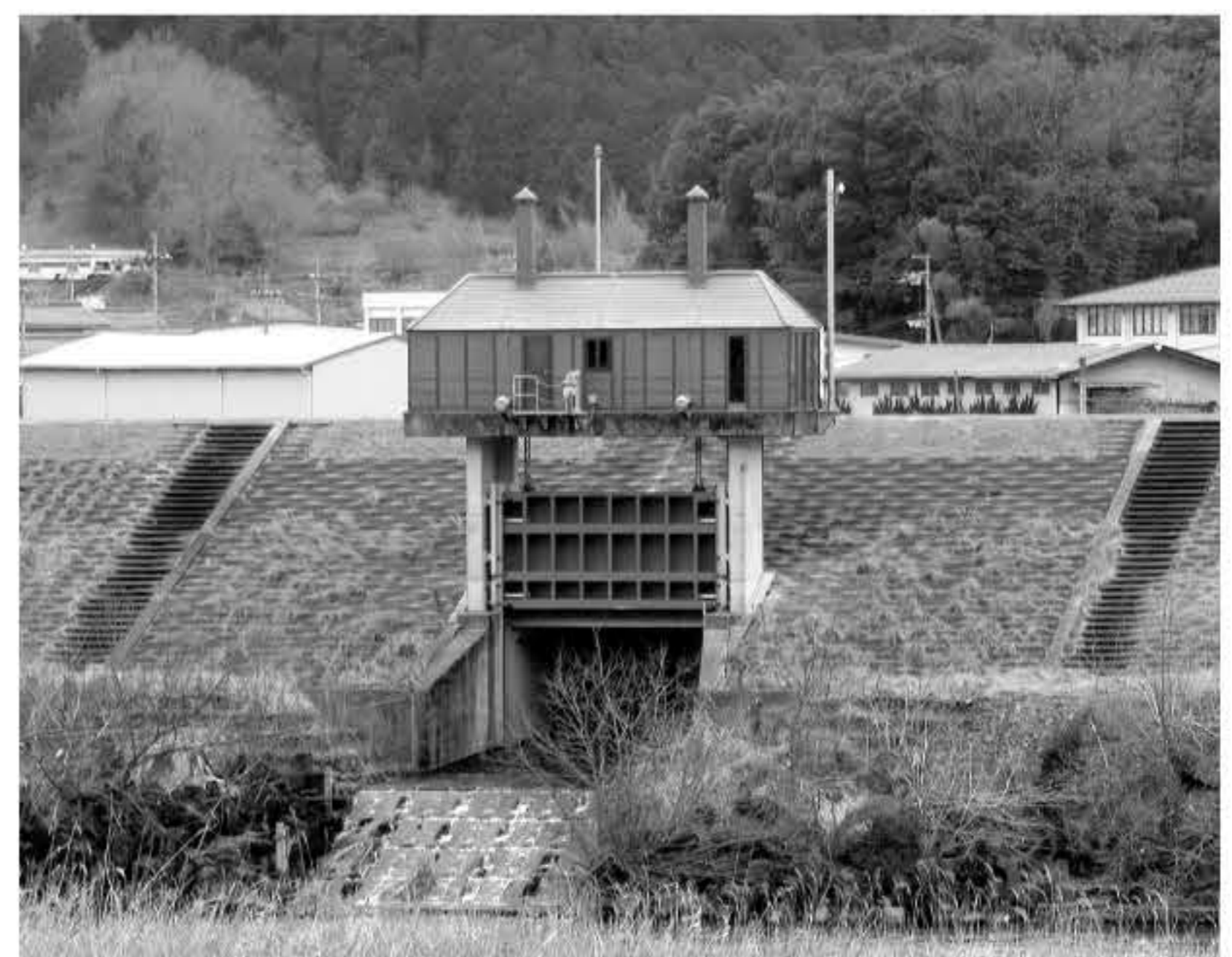
▲ 伊佐近隣の電動式樋門ゲート
