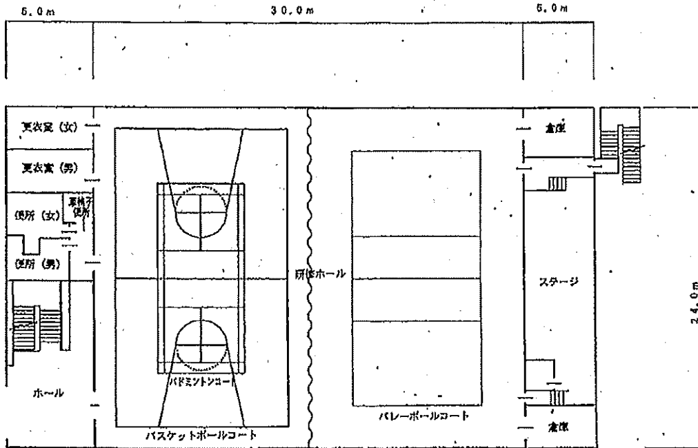
2階平面図
