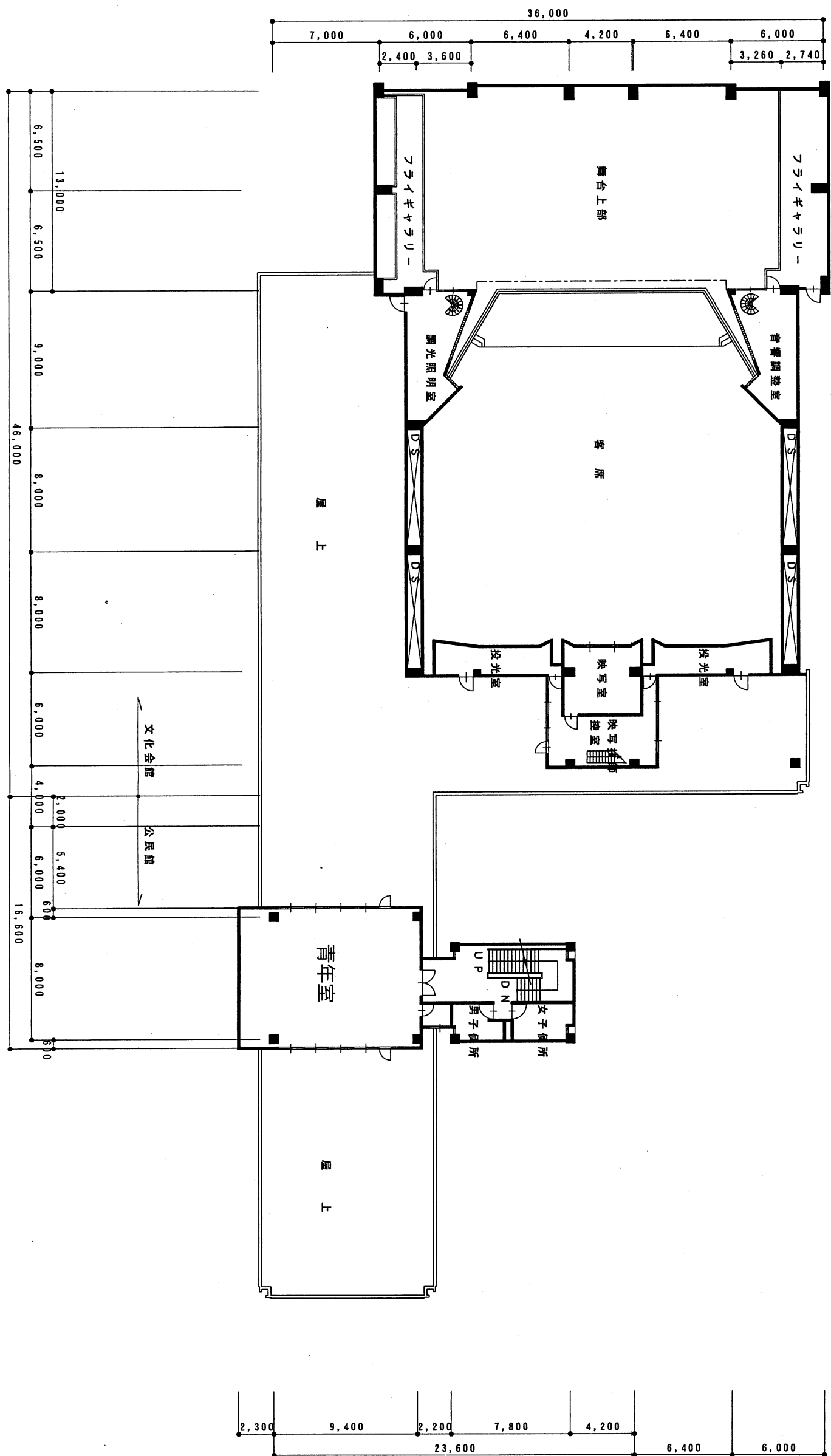
3階 平面図 S=1 /
