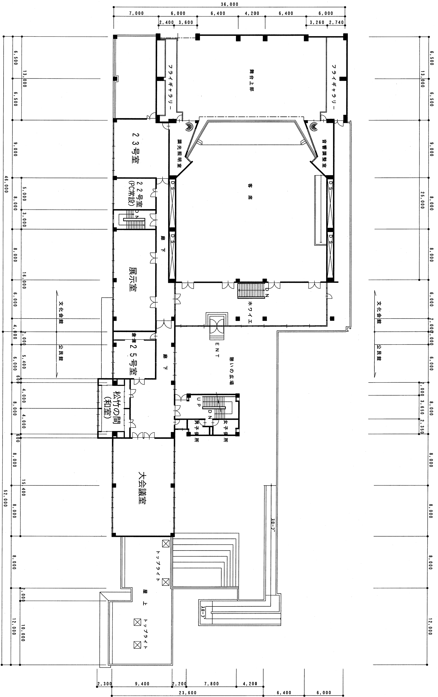
2階 平面図 S=1 /
